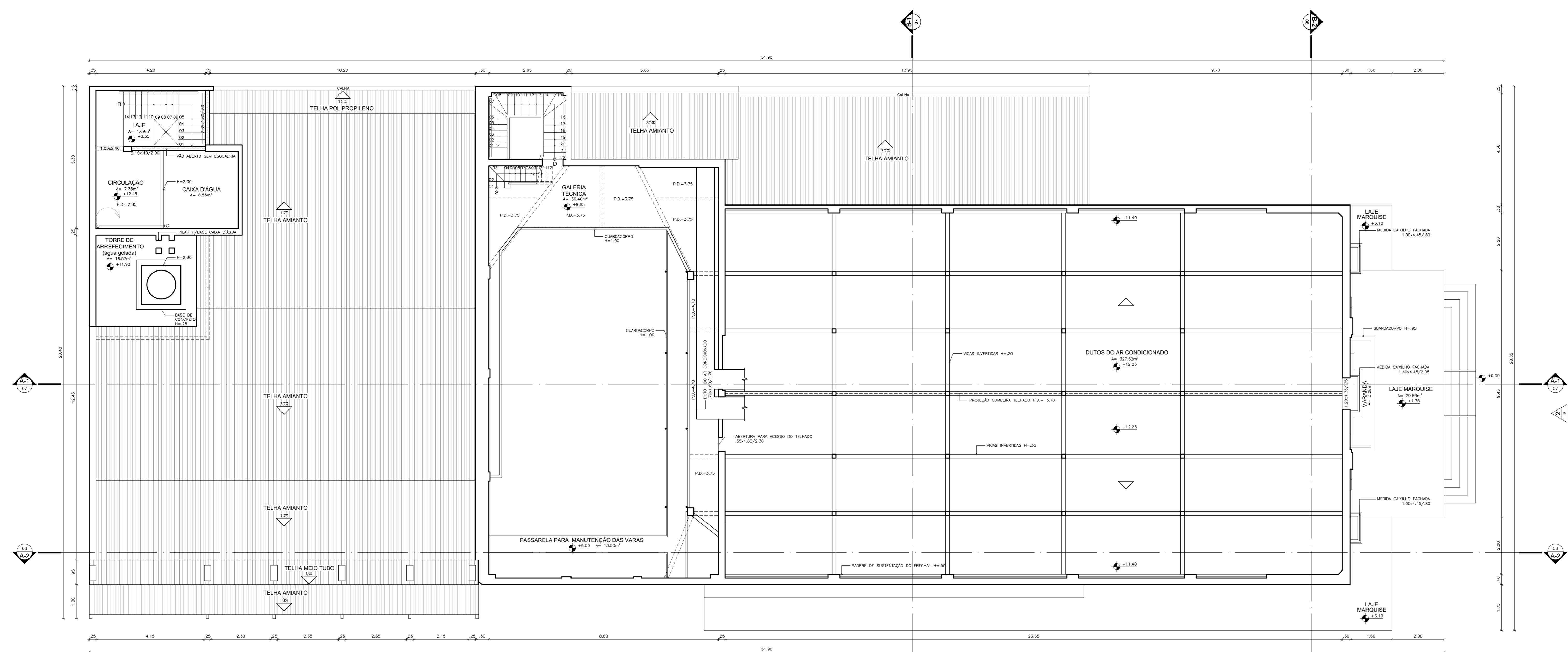
1 PLANTA BAIXA 3º PAVIMENTO
