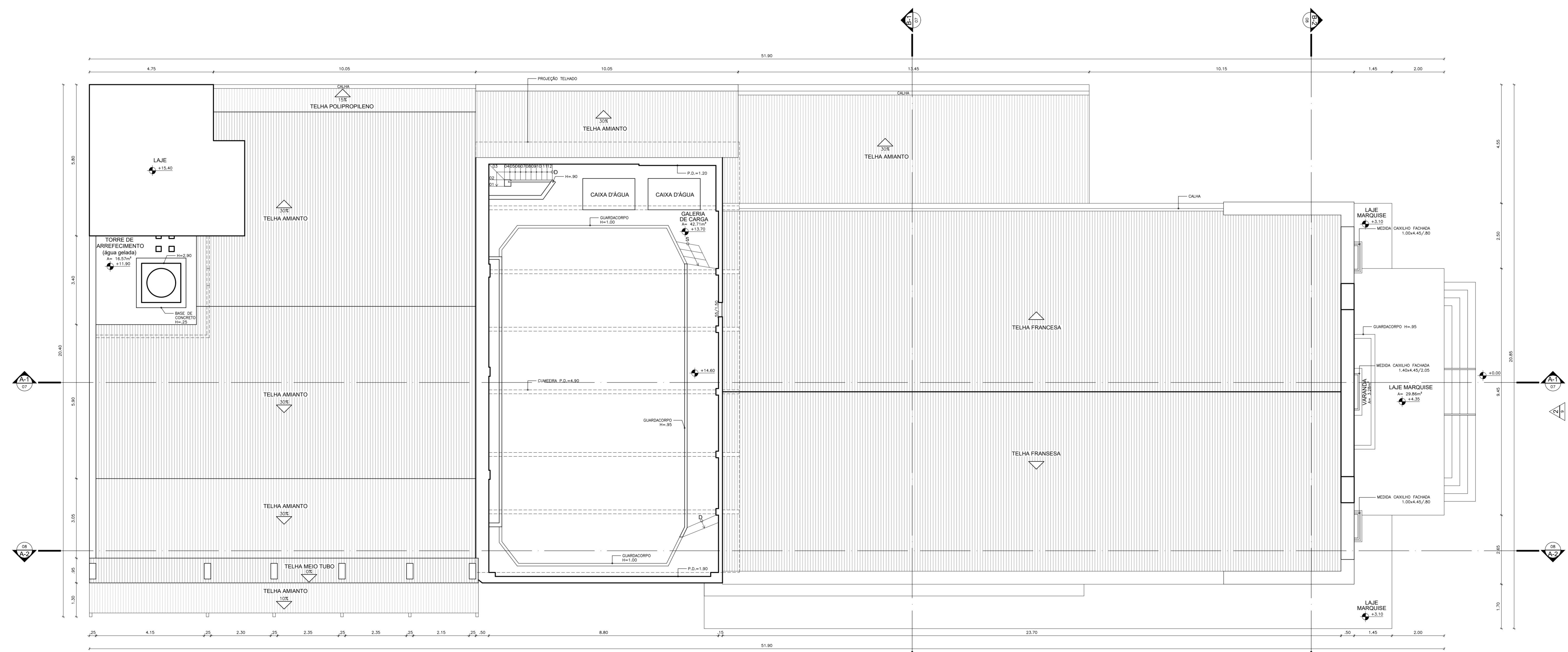
2 PLANTA BAIXA GALERIA DE CARGA
