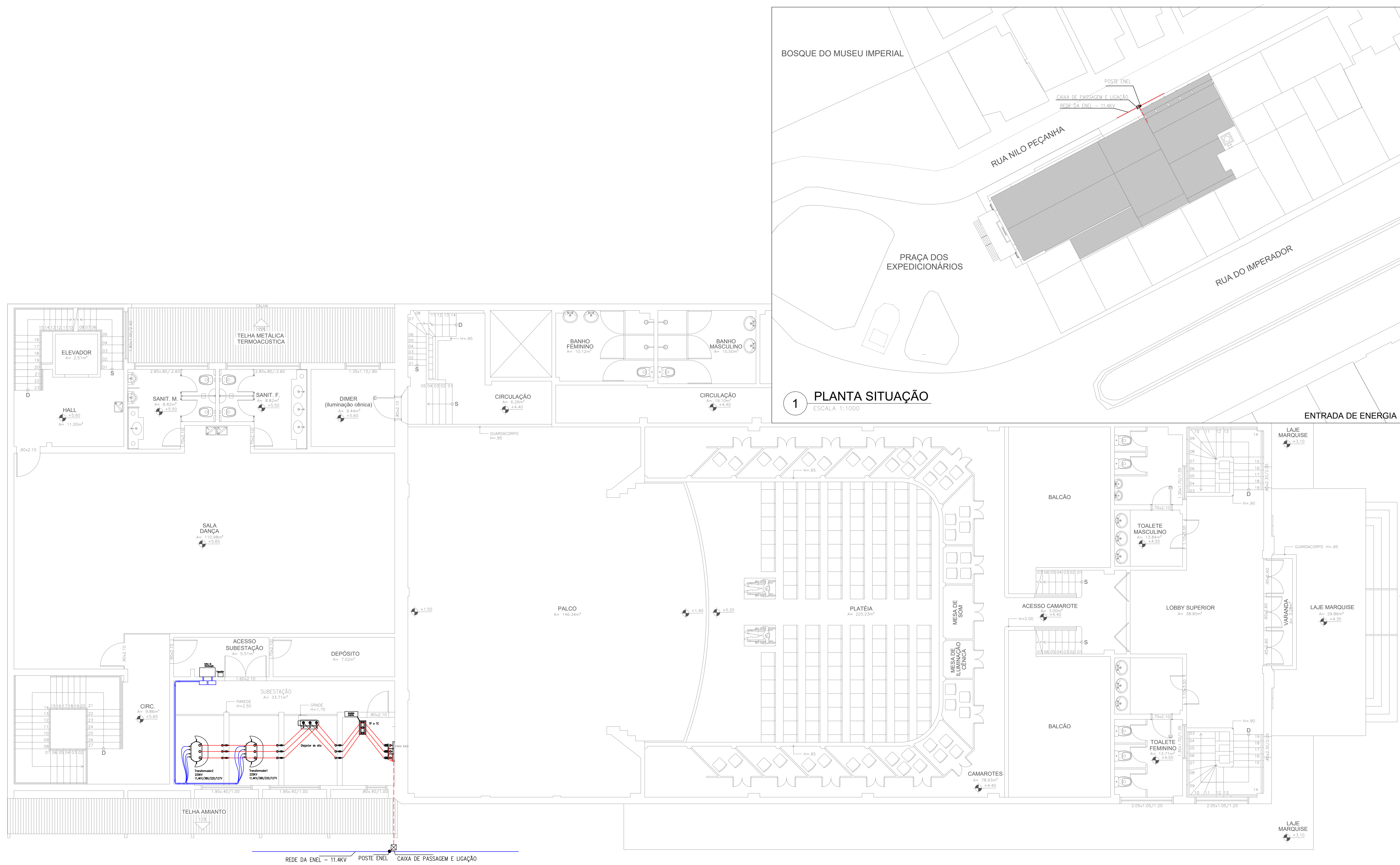
2 PLANTA BAIXA 1º PAVIMENTO - DETALHE ENTRADA DE ENERGIA ESCALA 1:50
