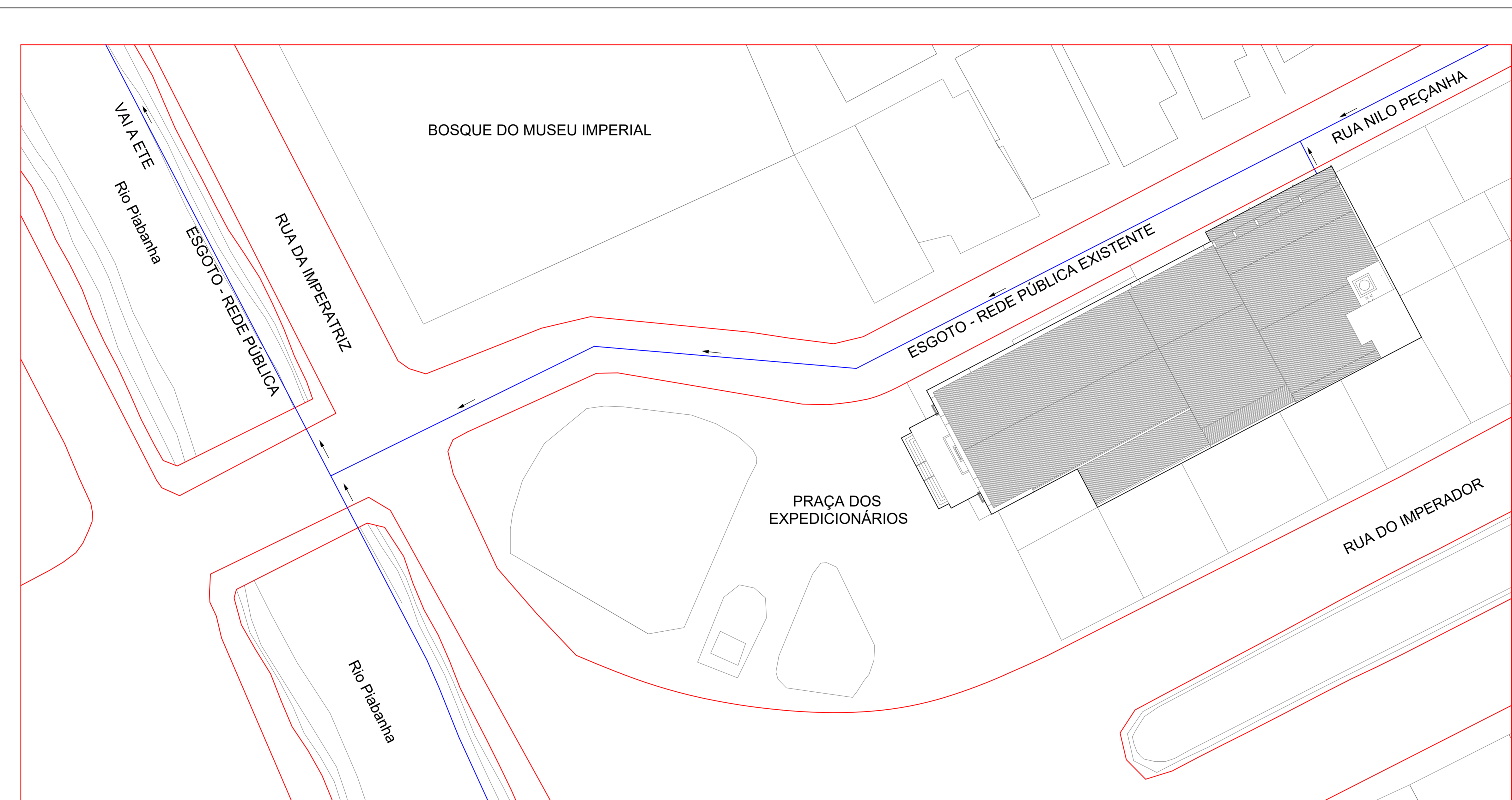
1 PLANTA SITUAÇÃO ESCALA 1:1000
