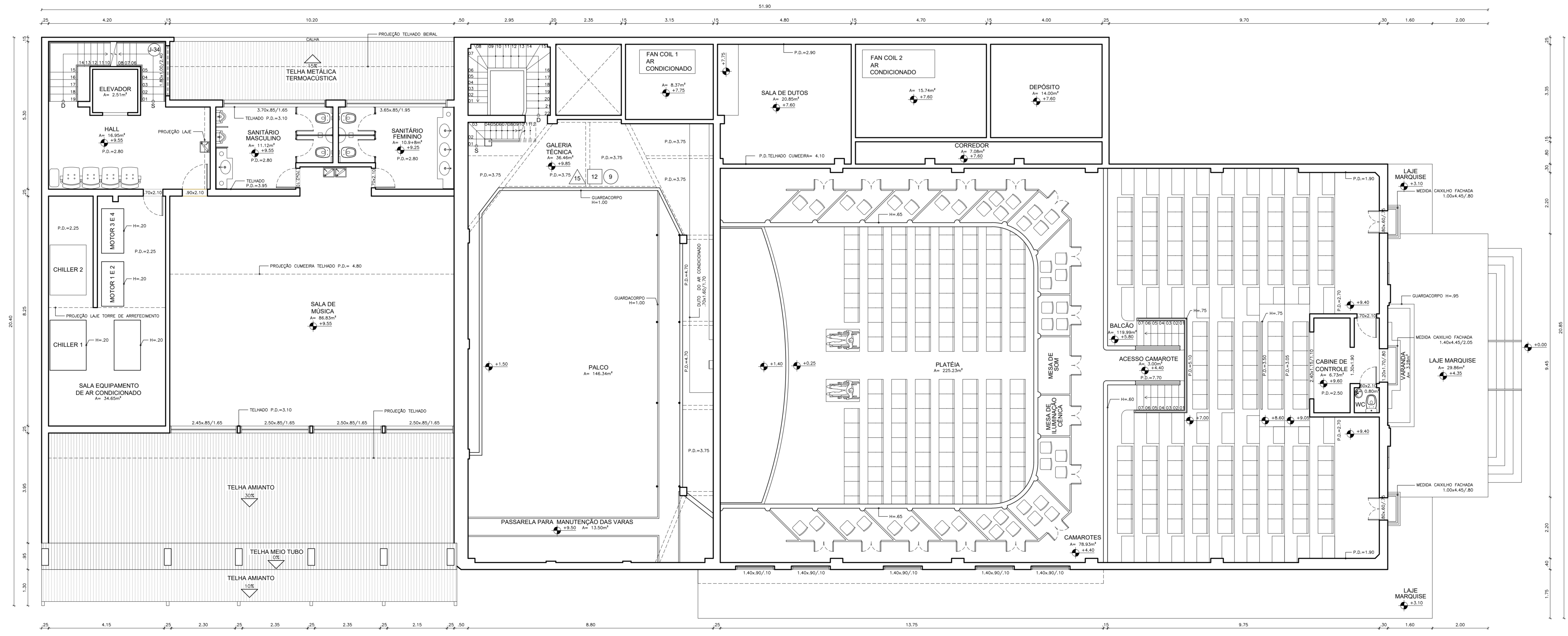
2 PLANTA BAIXA 2º PAVIMENTO
