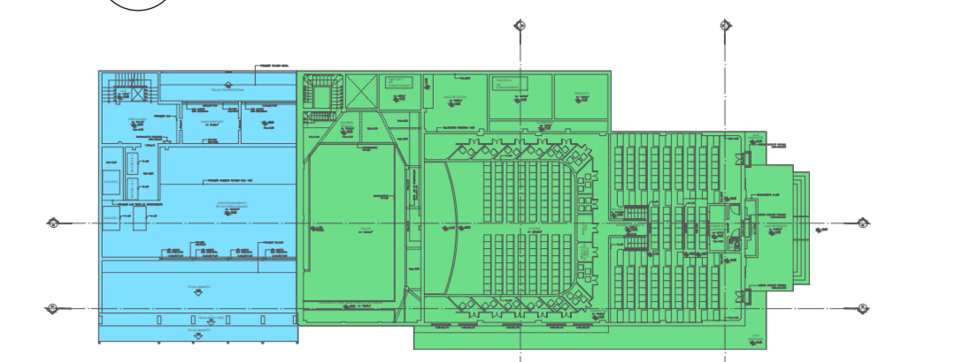
2 PLANTA BAIXA 2º PAVIMENTO
